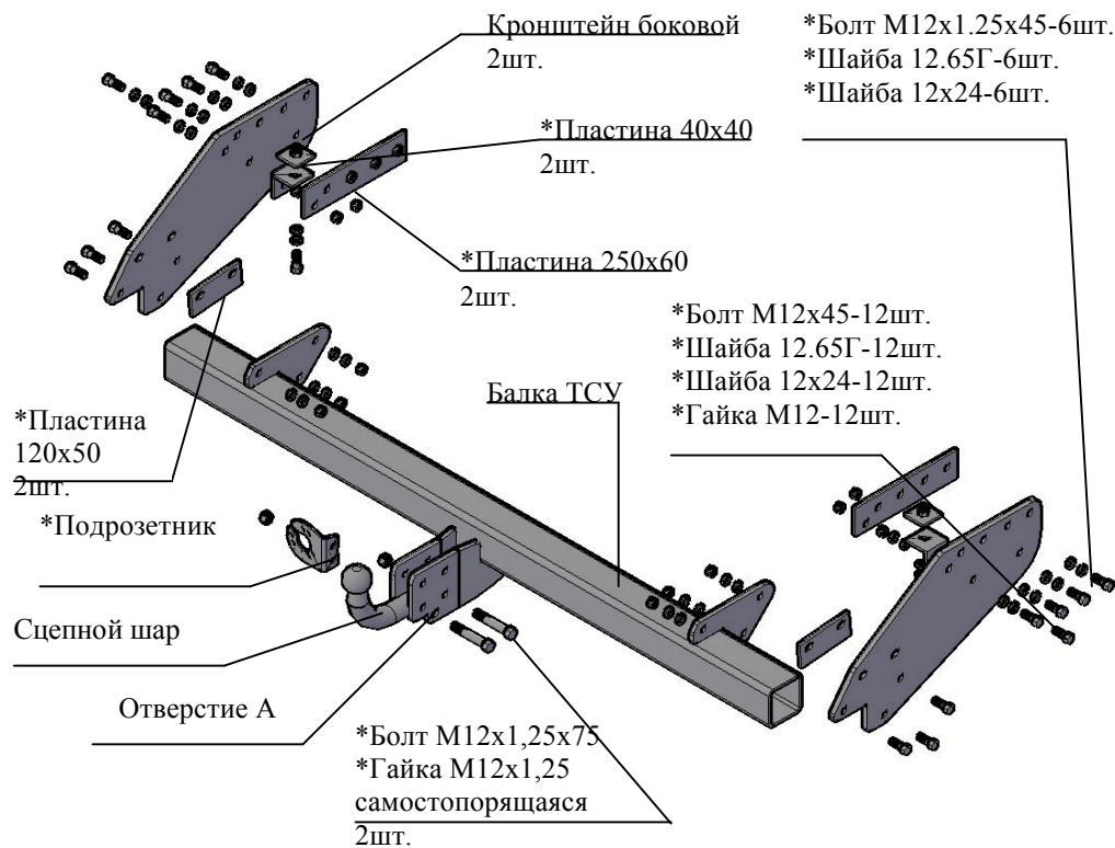
Рис.1 Тягово-сцепное устройство 7112
