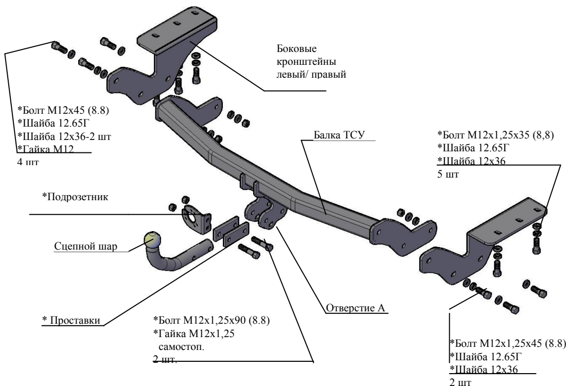
Рис.1 Тягово-сцепное устройство 7832.
